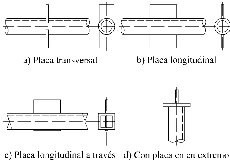
Figura C.1.2 Tipos de conexiones con placa
