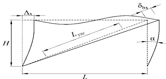
Figura 12.3.12 Deformación axial de los CRP
