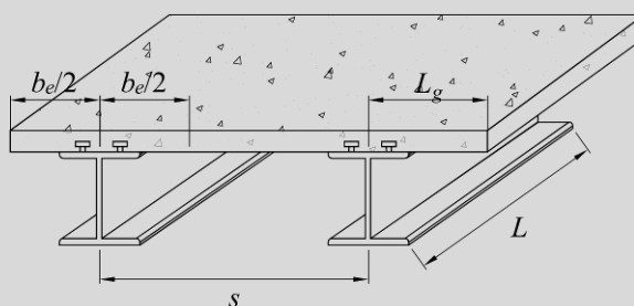
Figura 9.3.1 Ancho efectivo de vigas compuestas
