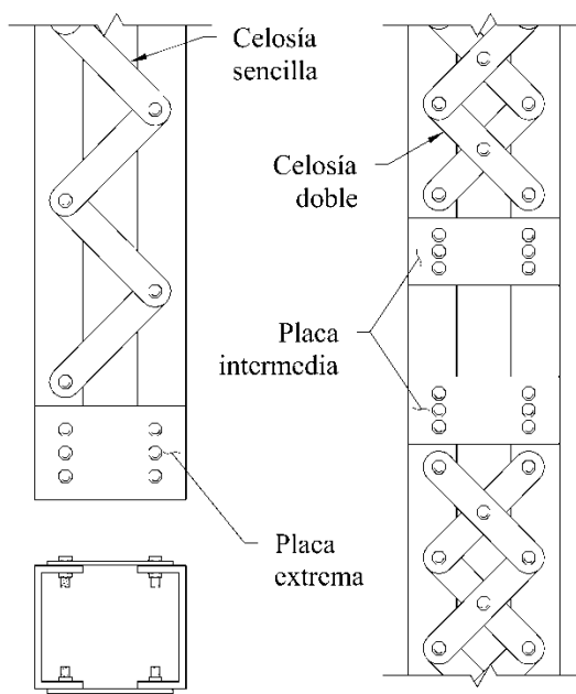
Figura 5.3.4 Celosías para armar miembros en compresión
