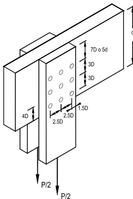
Figura 8.3.4 Espaciamento entre pernos de uniones con cargas perpendiculares a la fibra.
