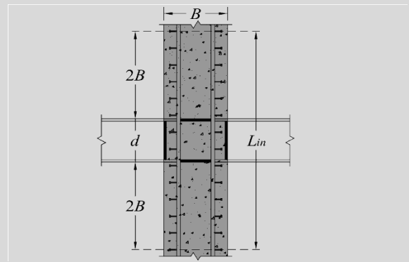
Figura 9.2.3 Longitud de introducción de la carga
