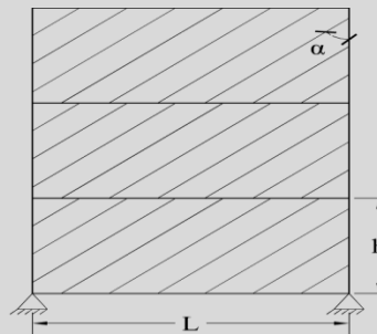
Figura 12.4.1 Modelo de franjas en unas placas de un TPD
