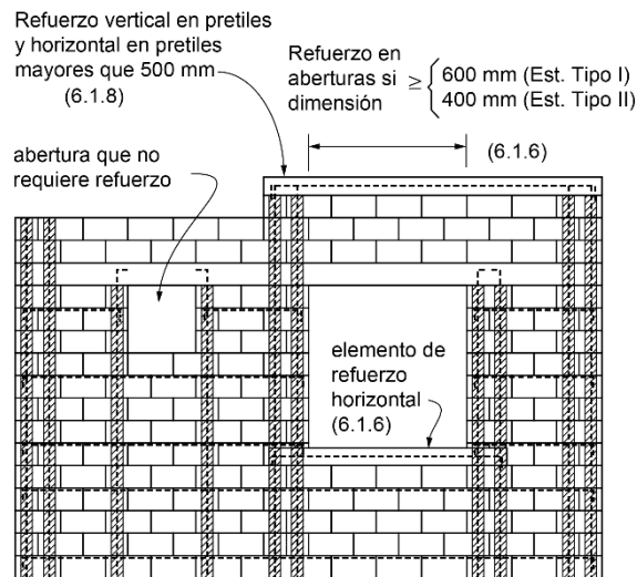
Figura 0.3 Refuerzo en aberturas y pretiles
